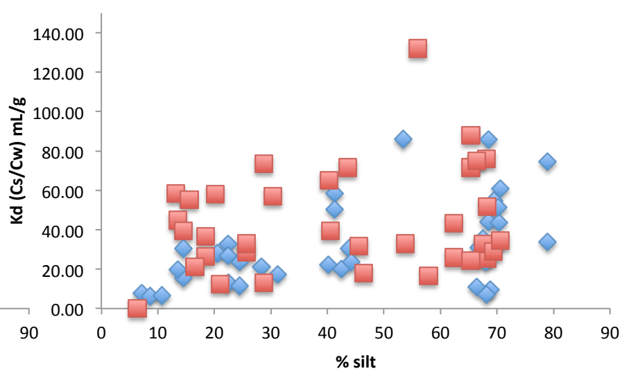
Kd vs. % silt
