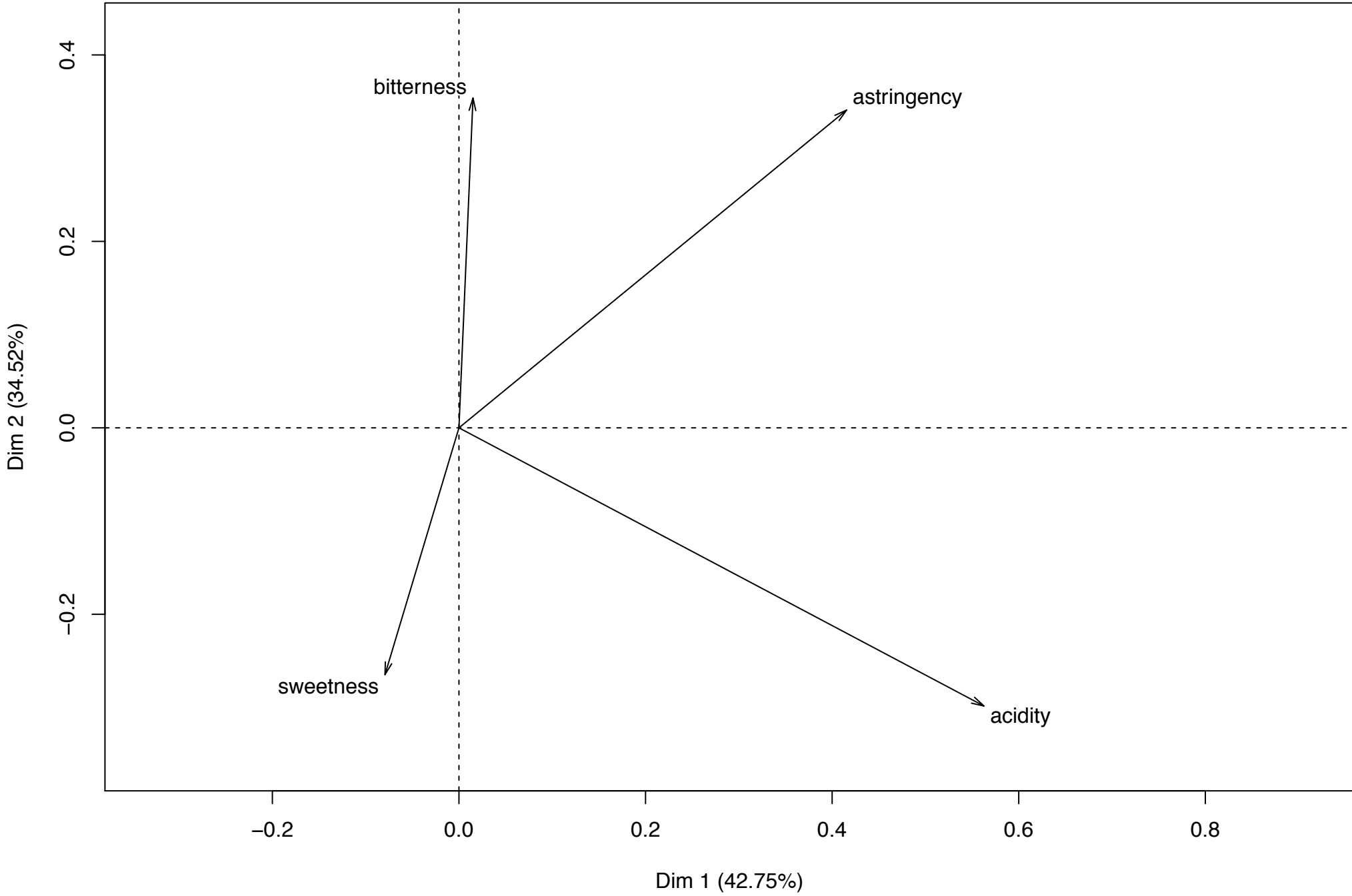
Variables factor map (PCA)
